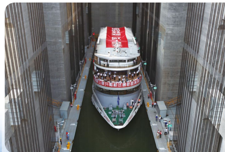
9 月 18 日下午，“长江三峡 9 号”客轮缓缓驶进三峡升船机。这标志着三峡工程建设的收官之作——三峡升船机正式进入试通航阶段。
