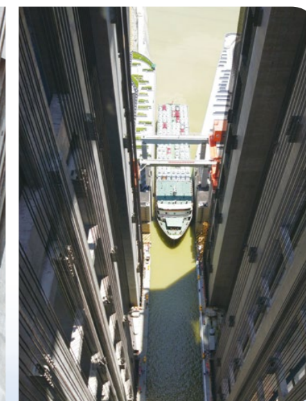
实船试航（进厢）
